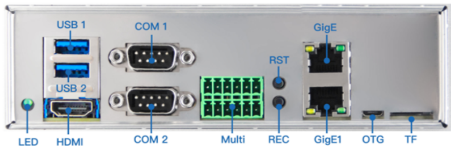
8F4E1 接口指示图
