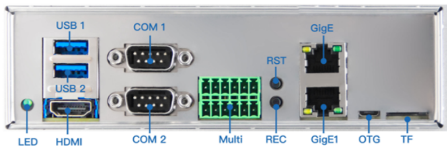
8F2E1 接口指示图
