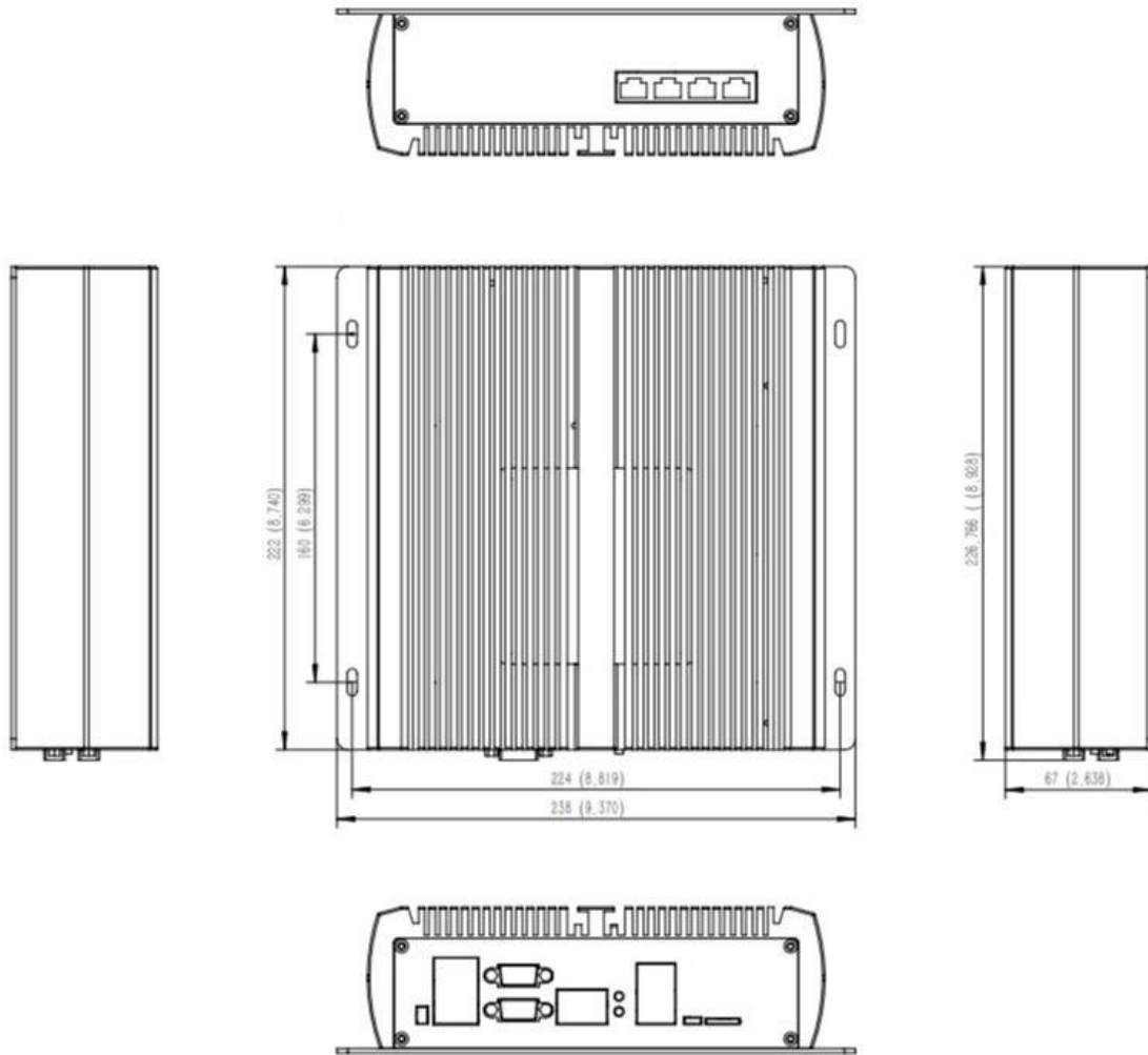
产品尺寸图
